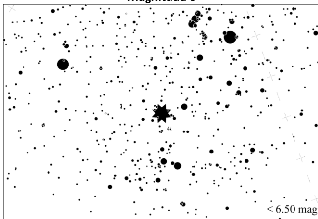
Magnituda 6
