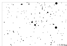
Peta Magnitudo 5
