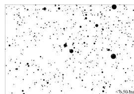
Peta Magnitudo 6
