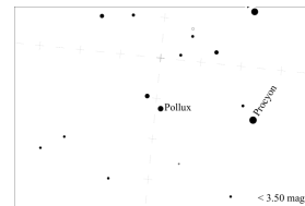
Peta Magnitudo 3
