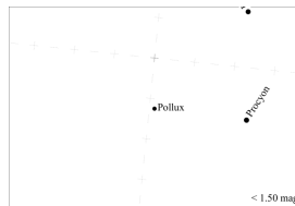
Peta Magnitudo 1
