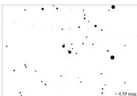
Peta Magnitudo 4
