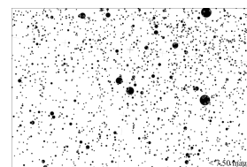
Peta Magnitudo 7
