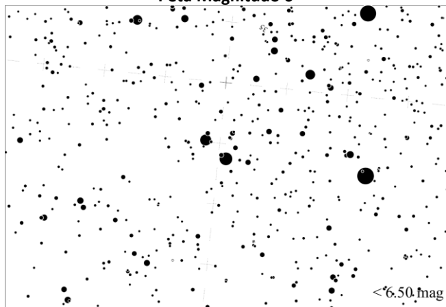
Peta Magnitudo 6
