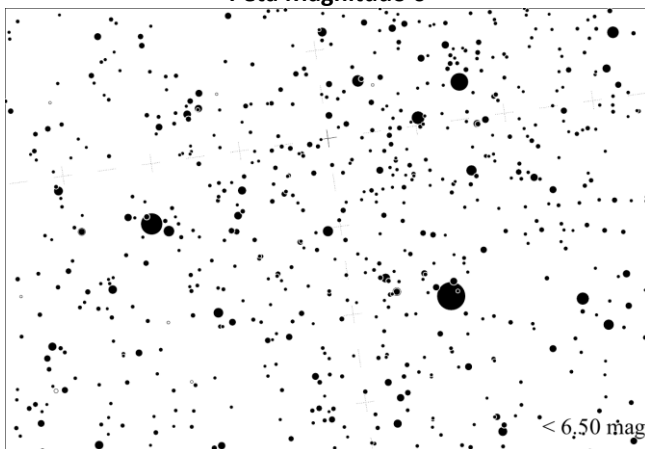
Peta Magnitudo 6
