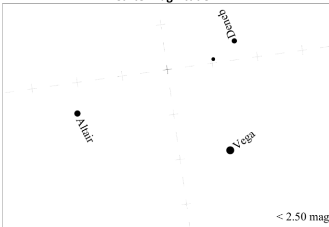
Carte Magnitude 2
